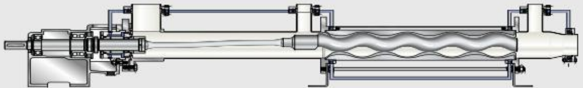
NEMO® SA Aseptic pump
