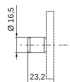
ALBERO D'ACCOPIAMENTO MOTORE MOTOR SHAFT CONNECTION
