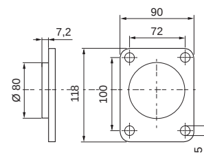
FLANGIA D'ACCOPIAMENTO MOTORE MOTOR FLANGE CONNECTION
